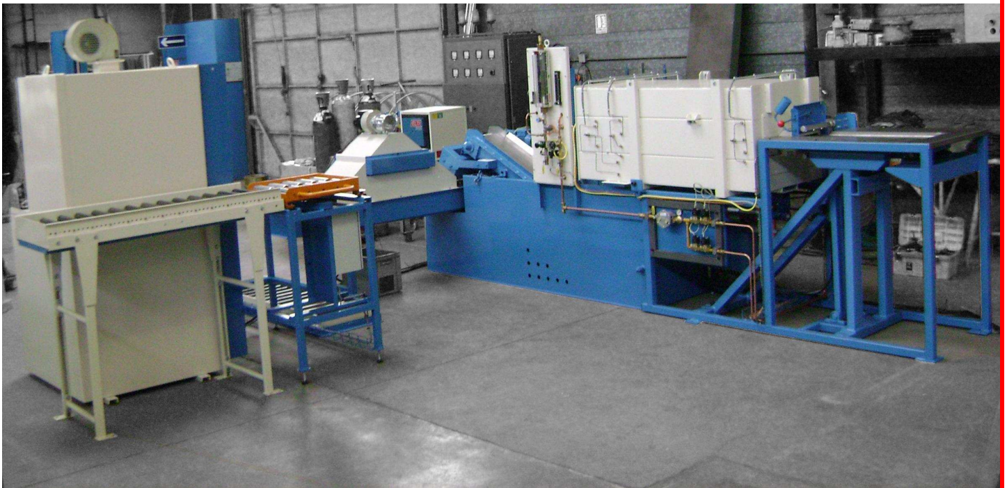
Ligne EASYSHAKE FSE 2 avec bac élévateur magnétique, démagnétiseur et ensemble de lavage + séchage Line EASYSHAKE FSE 2 with magnetic conveyor tank, degausser + washing and drying plant
